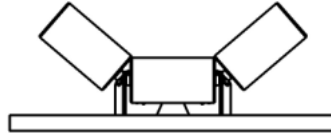
Variable Angle Sets – 20°, 30°, 40°, 50°, 60° Transome Type
